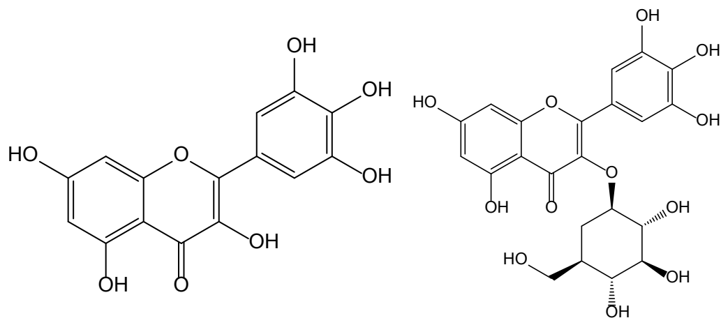
杨梅黄酮及其糖苷
