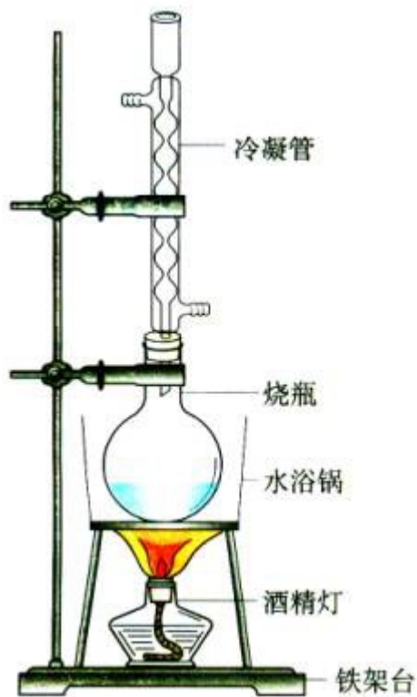
实验室热提取装置
